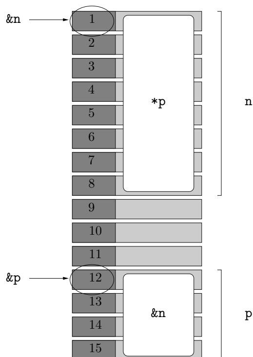
FIG. 5.1 – Relations entre une variable double n et un pointeur double *p=&n .
