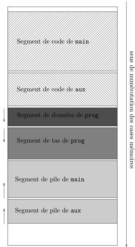
FIG. 3.1 – Schéma de l'organisation mémoire
