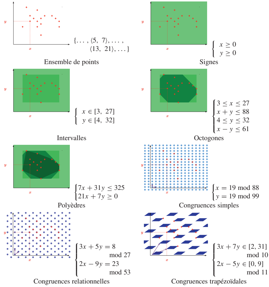
Figure 1. Approximations d'un ensemble de points
