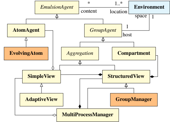
FIGURE 3 – Diagramme de classes de la hiérarchie des agents multi-niveaux dans le framework EMuLSion. Le comportement des agents de classes à fond orangé est contrôlé par une machine à états.
