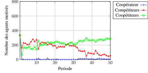
FIGURE 2 – L’évolution de la performance d’une plateforme homogène
