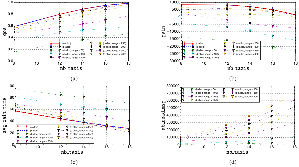
FIGURE 4 – Qualité de service (4a), gain (4b), temps moyen d’attente d’un client (4c) et nombre de messages lus par des taxis (4d) pour les différentes stratégies avec des rayons de commmunication pour la stratégie décentralisée en utilisant des interactions P2P, pour un nombre croissant de taxis.
