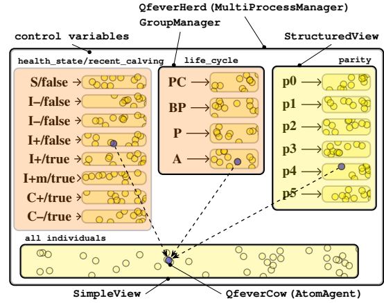
FIGURE 7 – Structure du modèle intra-troupeau de la fièvre Q. Les individus sont rassemblés en fonction des valeurs des variables clefs de chaque aspect du modèle. On accède aux individus (e.g. celui représenté en bleu, dans l’état de santé I^+ , le cycle de vie A et de parité 4) soit par aspect, soit par l’agent SimpleView hébergeant tous les atomes.
